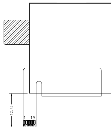
FPC弯折示意图 FPC弯折出货
