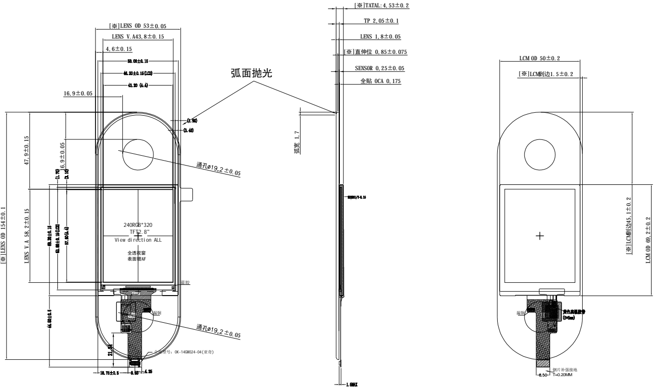
正视图
