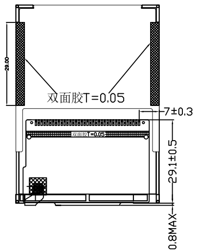
FPC弯折后客户参考图 展开出货
