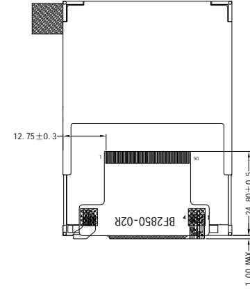
FPC弯折示意图 FPC展开出货
