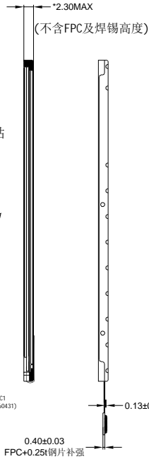
侧视图
