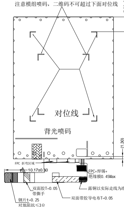
背视图
