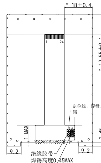
弯折示意图 FPC弯折粘贴出货
