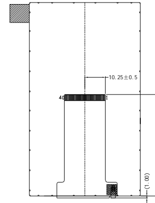
FPC弯折示意图 FPC弯折出货
