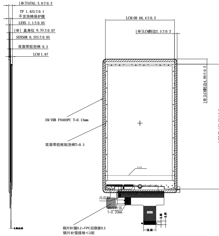
侧视图
