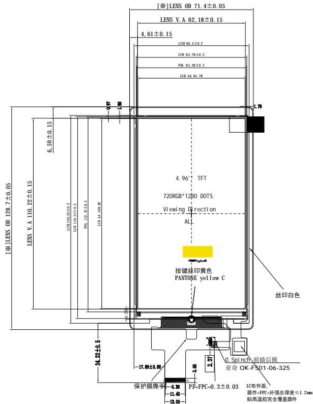
正视图
