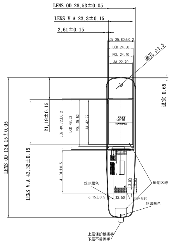
正视图
