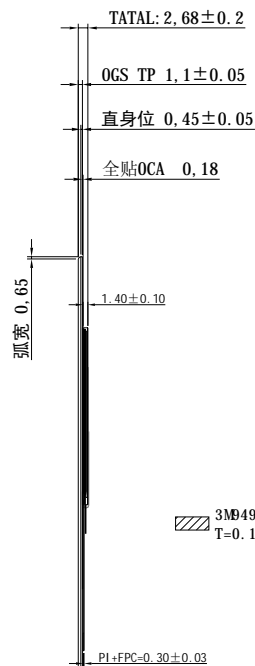
侧视图
