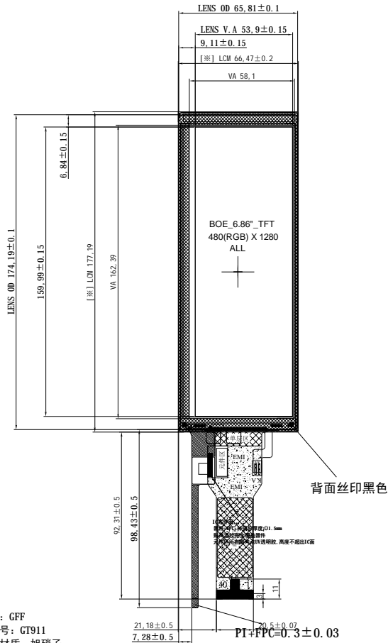
正视图
