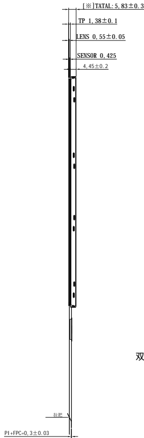
侧视图
