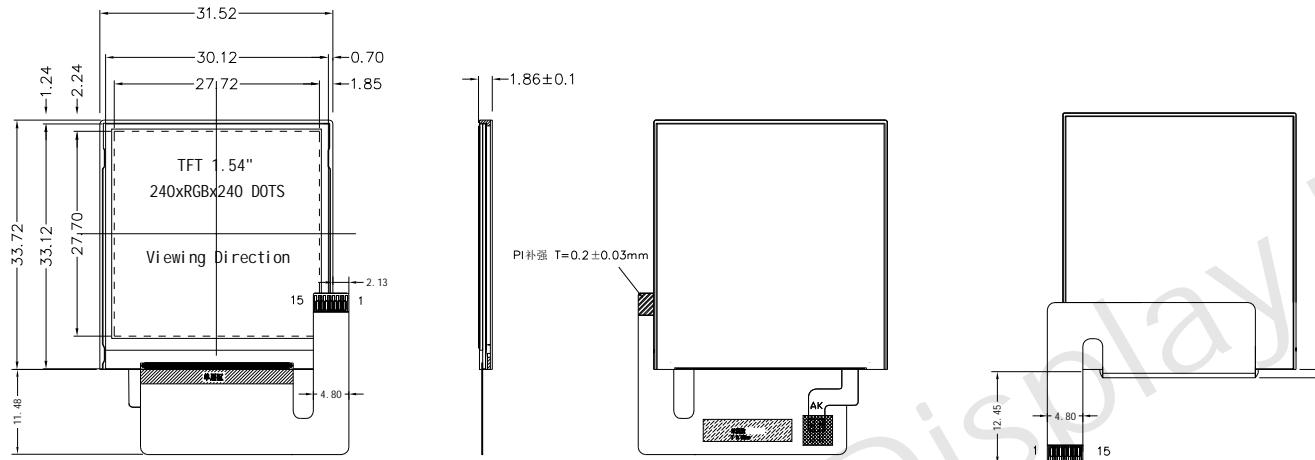
FPC弯折后客户参考图
