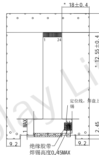
弯折示意图 FPC弯折粘贴出货
