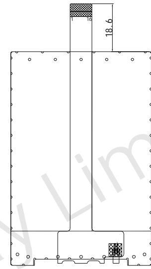
FPC弯折示意图 FPC弯折出货
