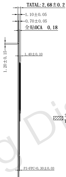
侧视图
