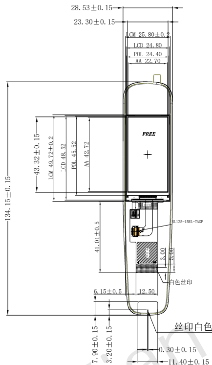
正视图
